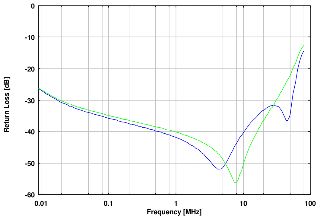
Abb. 2 Anpassung des SY9223-150 (EuT mit 150 \Omega abgeschlossen) Fig. 2: Return loss of SY9223-150 (EuT terminated with 150 \Omega )
