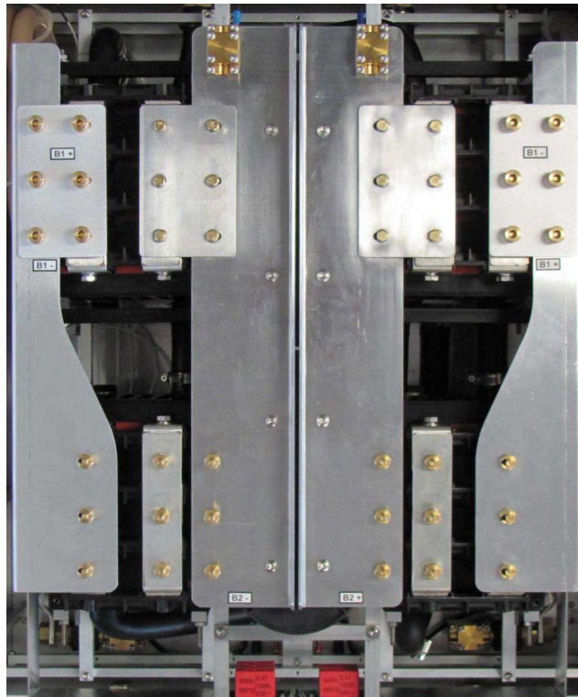
Abb. 7. Konfigurationsbeispiel für 2 x ( R_{int} = 50 \text{ m}\Omega ). Brücke B1 ist eingesetzt. (Brücken B1, B3 sind nicht installiert).
