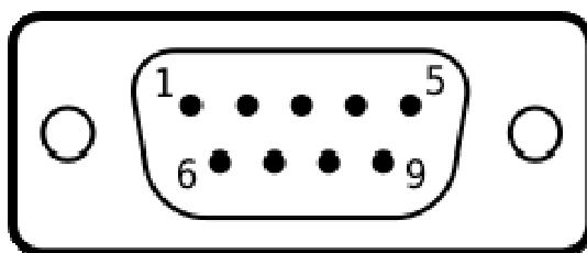
Abb. 9. D-SUB-Stecker, Sicht von vorne. Fig. 9. D-SUB-plug, front view.
