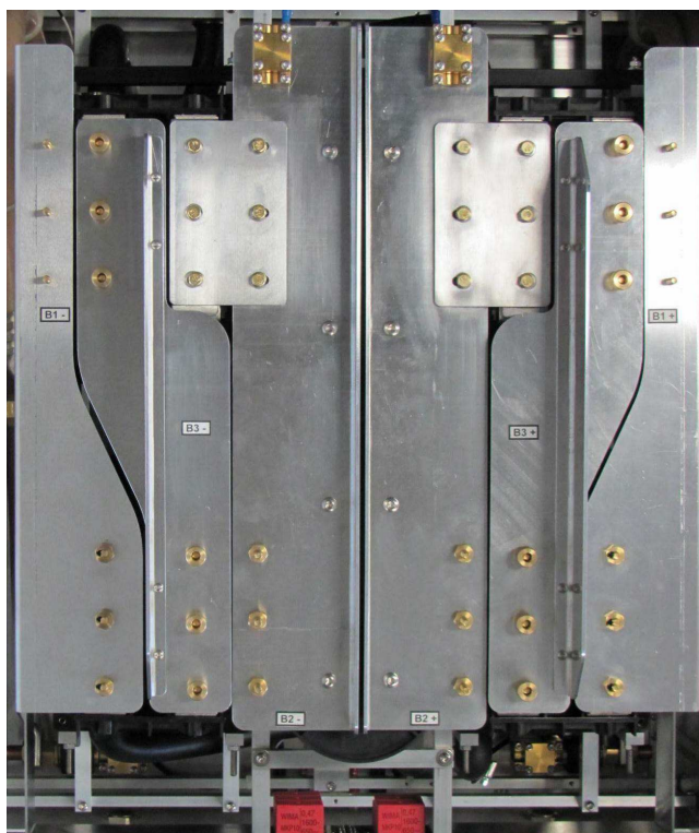
Abb. 6. Konfigurationsbeispiel für 2 x ( R_{int} = 100\text{ mOhm} ). Brücke B3 ist eingesetzt. (B1 und B2 sind nicht installiert).
