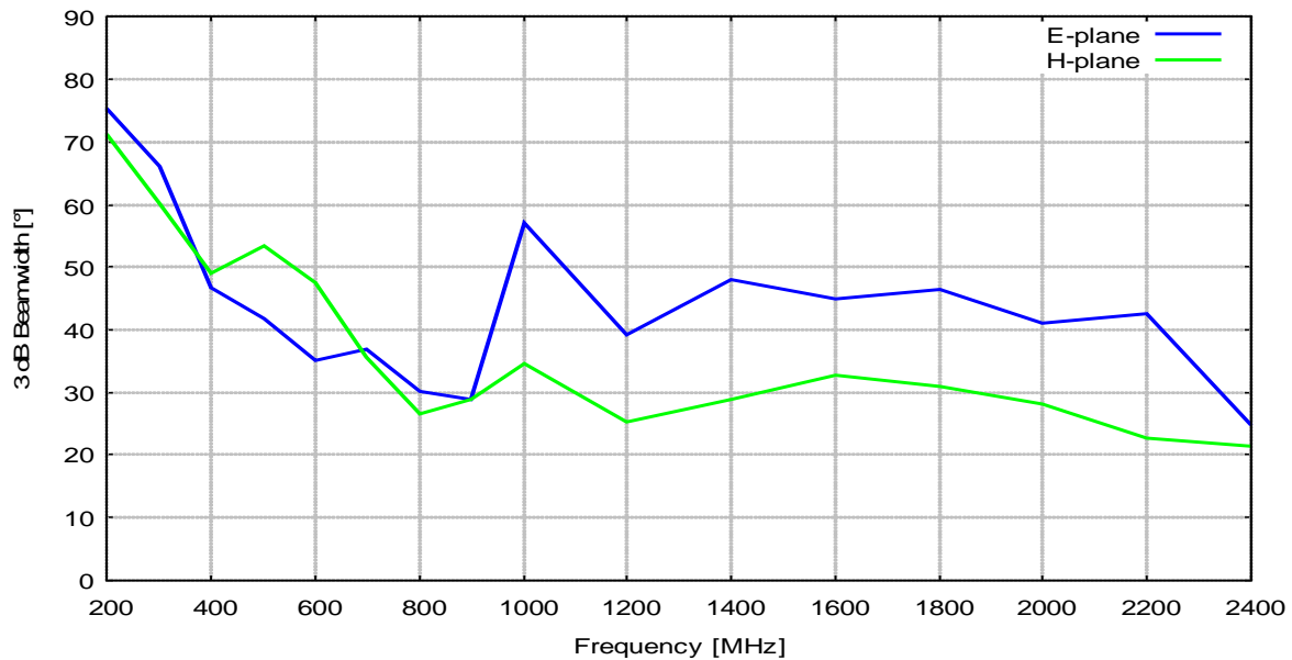
3 dB Öffnungswinkel
