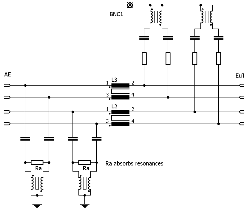
Bild 7: Prinzipschaltbild CDN T4 4A Fig. 7: Circuitry CDN T4 4A
