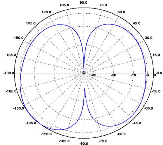
H-Ebene / H-Plane 310 MHz
