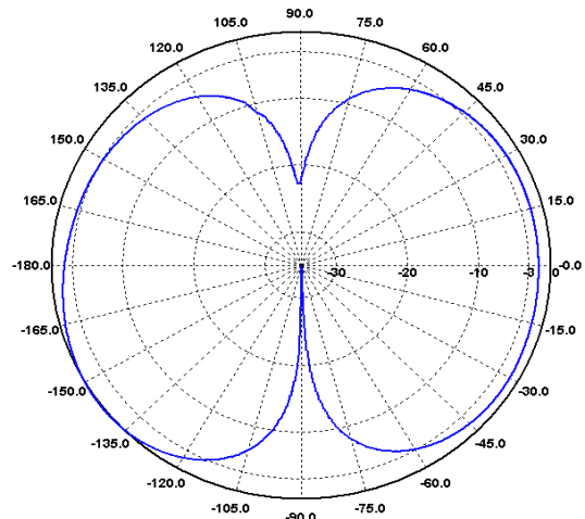
H-Ebene / H-Plane 240 MHz
