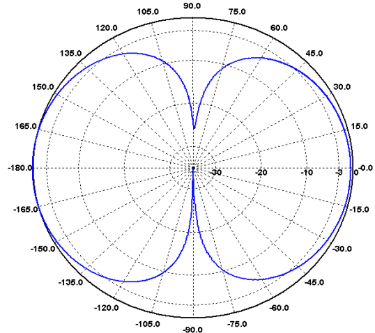
H-Ebene / H-Plane 190 MHz
