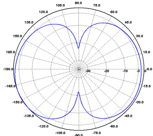
H-Ebene / H-Plane 230 MHz
