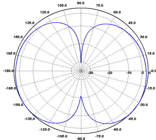
H-Ebene / H-Plane 260 MHz
