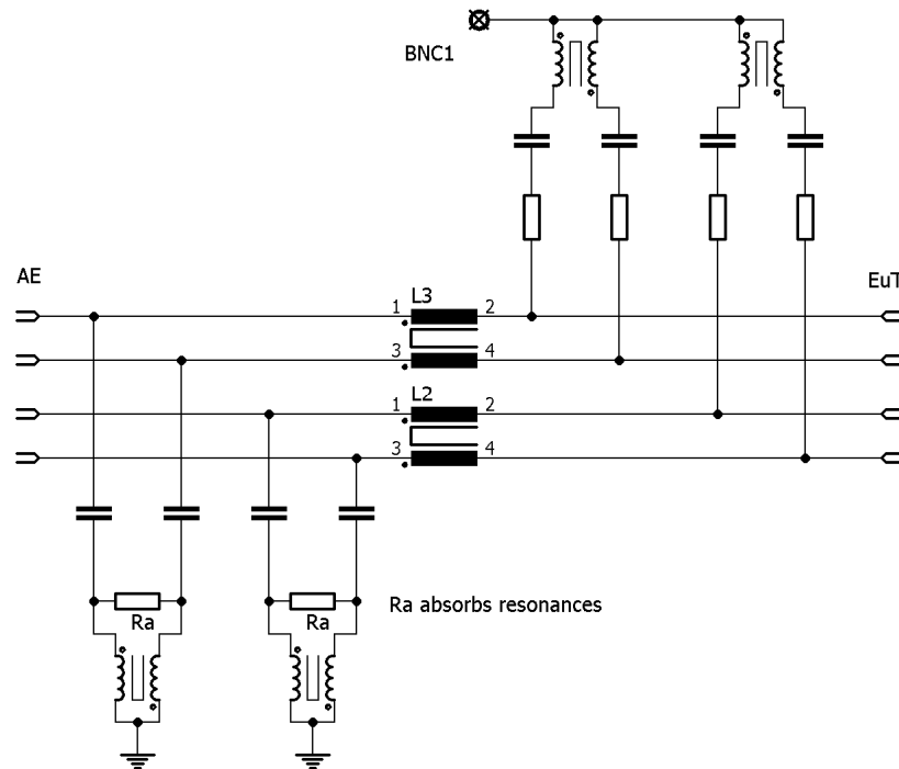
Bild 7: Prinzipschaltbild CDN T4 Fig. 7: Circuitry CDN T4
