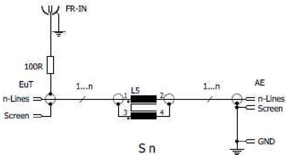
Bild 4: Prinzipschaltbild CDN S25 SUBD Fig. 4: principal circuitry CDN S25 SUBD
