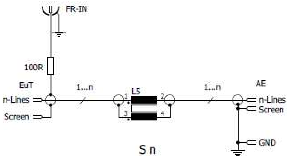
Bild 3: Prinzipschaltbild CDN S25 SUBD Fig. 3: principal circuitry CDN S25 SUBD
