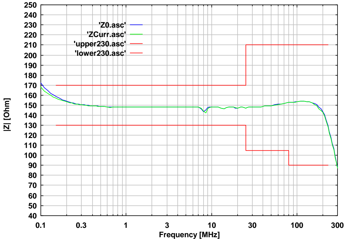
Bild 1: typ. EuT Gleichtaktimpedanz mit und ohne Laststrom Fig. 1: typ. EuT Common mode impedance
