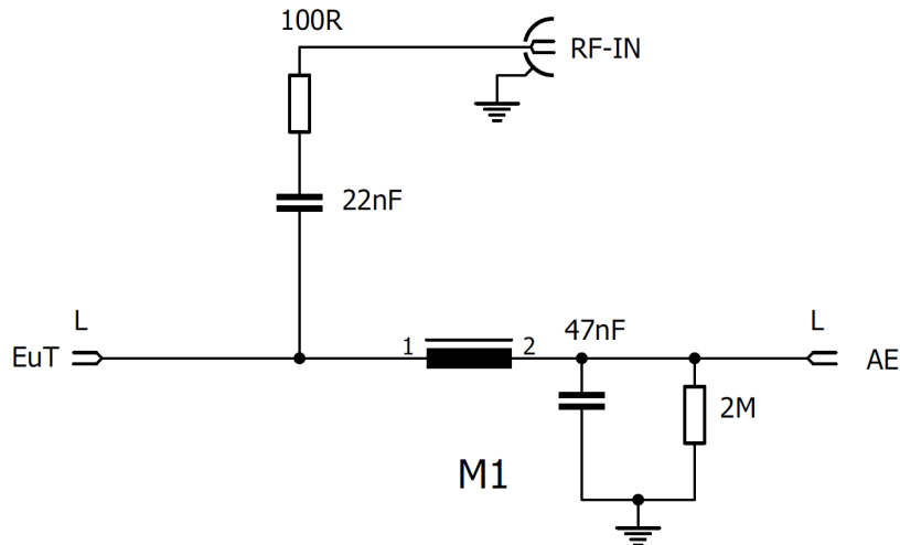
Bild 5: Prinzipschaltbild CDN M1 16A 1000V Fig. 5: principal circuitry CDN M1 16A 1000V
