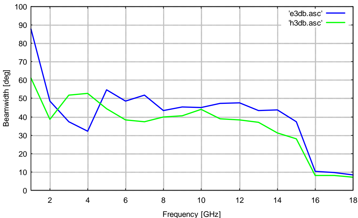
3 dB Beamwidth
