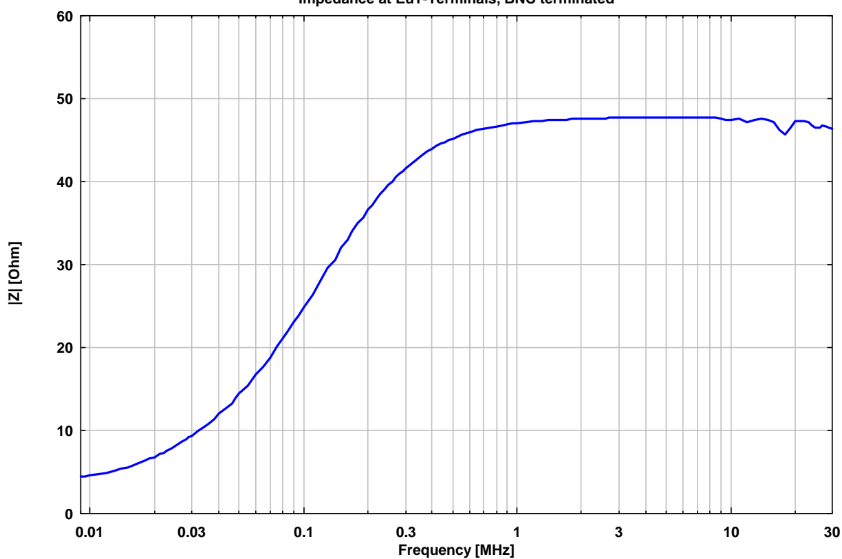
Impedanz an den Prüflingsklemmen, BNC mit 50 Ω Abschluss Impedance at EuT-Terminals, BNC terminated
